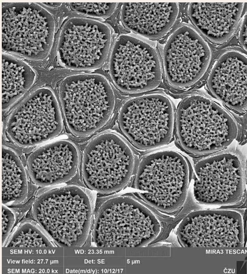
Ve ztenčeninách buněčné stěny jsou vidět zrnka oxidu křemičitého, které zcela ucpávají cévu dřeviny meranti ( Shorea spp. ). Radiální řez, zvětšeno 20 000krát.
