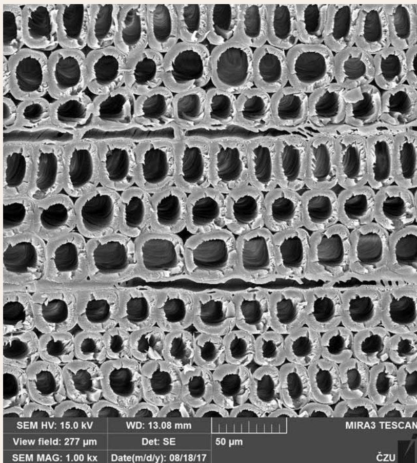
Příčný řez smrkovým dřevem, který při 1 000násobném zvětšení zobrazuje tracheidy reakčního tlakového dřeva s okrouhlým průřezem, tlustou buněčnou stěnou a nápadně velkými mezibuněčnými prostory.
