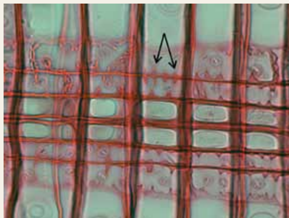
Zubaté ztluštění v cévích dřevových paprsků borovice lesní. Radiální řez, zvětšeno 400krát.
