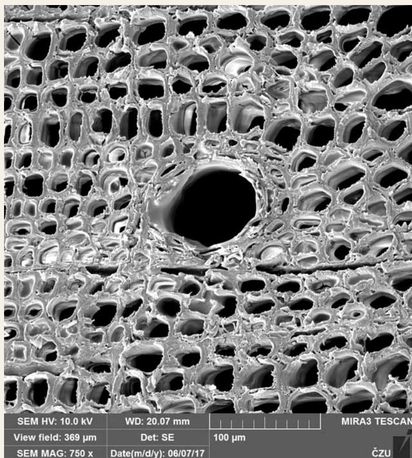
Vertikální pryskyřičný kanálek na příčném řezu borovice při 750násobném zvětšení.
