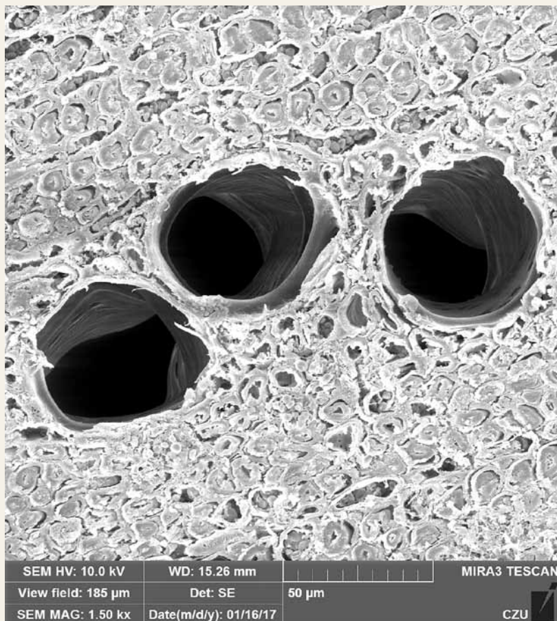
Kruhovitě pórovitá stavba dubu.
