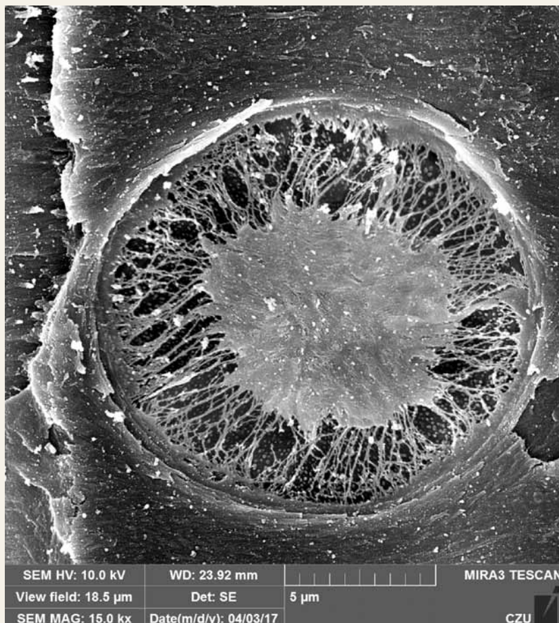
Fotografie dvojtečky, „přírodního uzavíracího ventilu“, pořízená elektronovým mikroskopem při 15 000násobném zvětšení.
