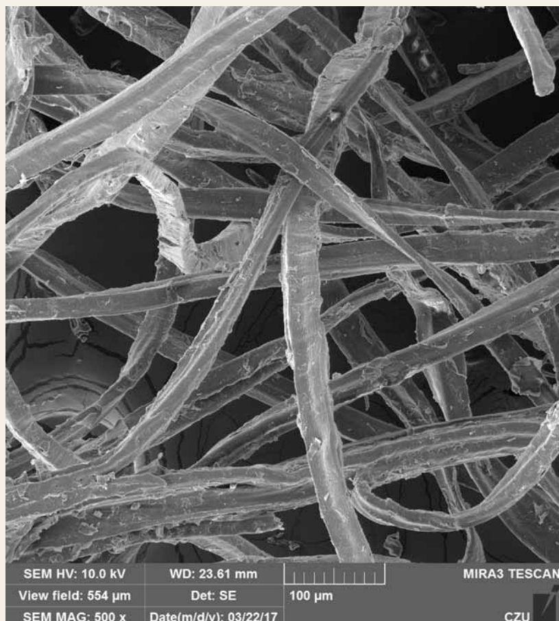
Snímek z elektronového mikroskopu zobrazuje 500× zvětšené tracheidy, označované nikoli bezdůvodně jako vlákna. Rozvláknění dřeva bylo provedeno pomocí defibrátoru při teplotě 180 °C.
