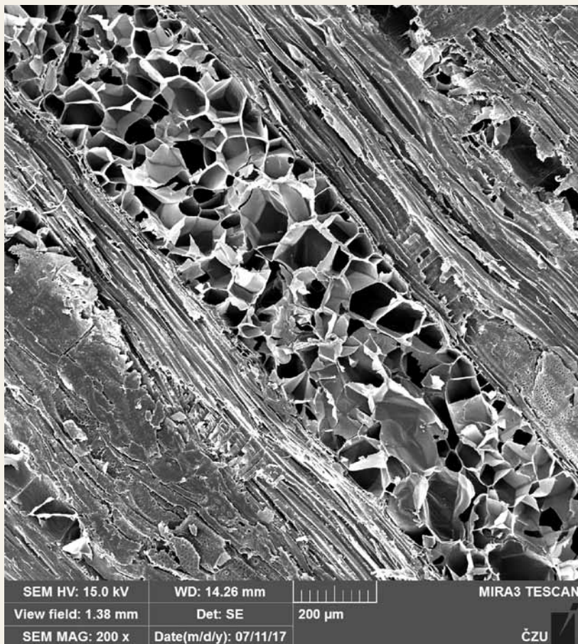
Na mikroskopickém snímku je při 200násobném zvětšení zobrazen podélný řez dřevem akátu. Uhloučkou snímku tvoří céva, na které je patrné její kompletní ucpání thylami.
