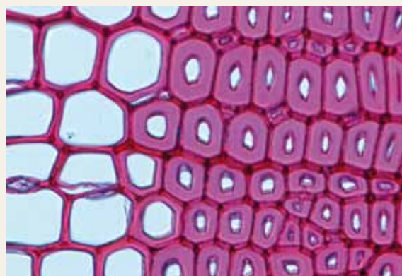
Příčný řez dřevem modřínu opadavého, zvětšeno 600×. V levé části obrázku se nachází tenkostěnné jarní tracheidy, v pravé části tlustostěnné letní tracheidy.
