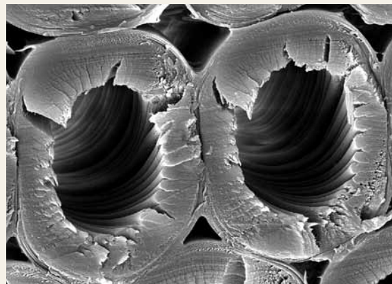
Detail tracheid reakčního tlakového dřeva s velkým odklonem lamel celulózy od podélné osy buňky, jenž způsobuje větší sesychání v podélném směru. Zvětšeno 5 000krát.
