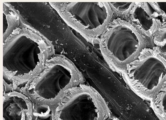
Příčný řez dřevem cedru zobrazuje dřevěný paprsek, který vede od středu kmene směrem k obvodu narušuje jinak zcela kompaktní strukturu tvořenou tracheidami.
