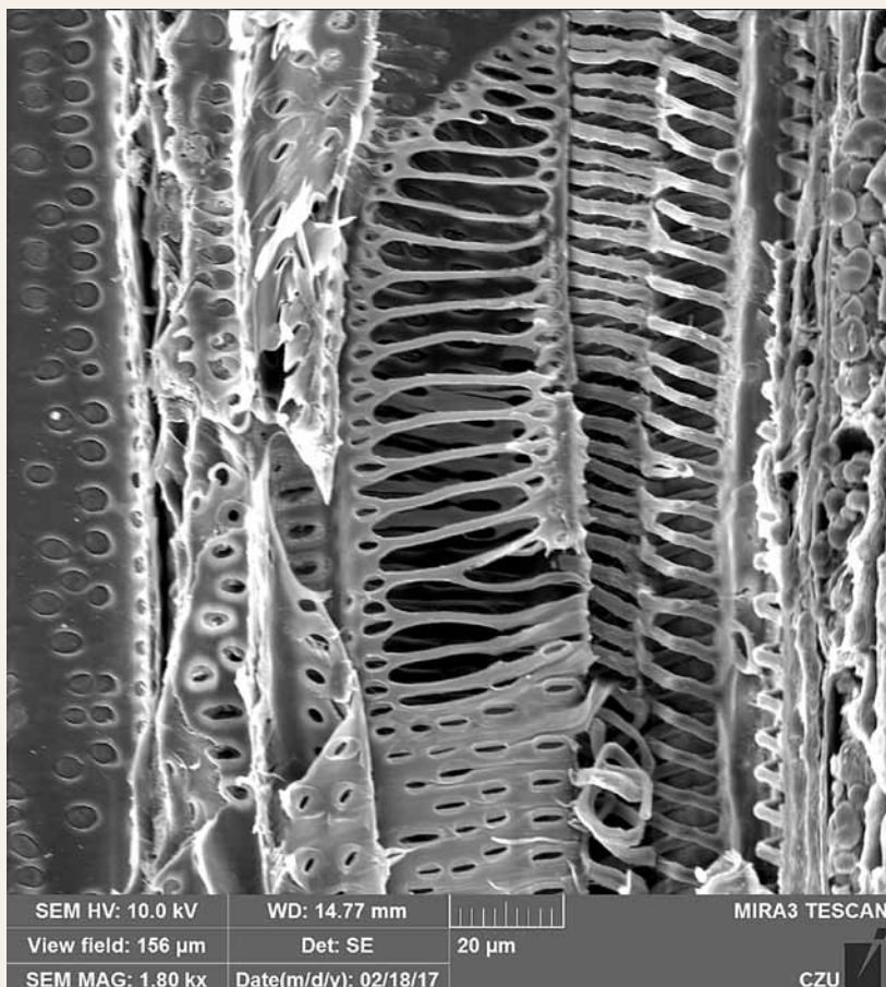
Na středu snímku je zobrazena žebříčkovitá perforace příčné přehrádky mezi dvěma cévními články. Toto propojení cévních článků umožňuje vedení vody ve vertikálním směru. Fotografie byla pořízena elektronovým mikroskopem při zvětšení 1 800.
