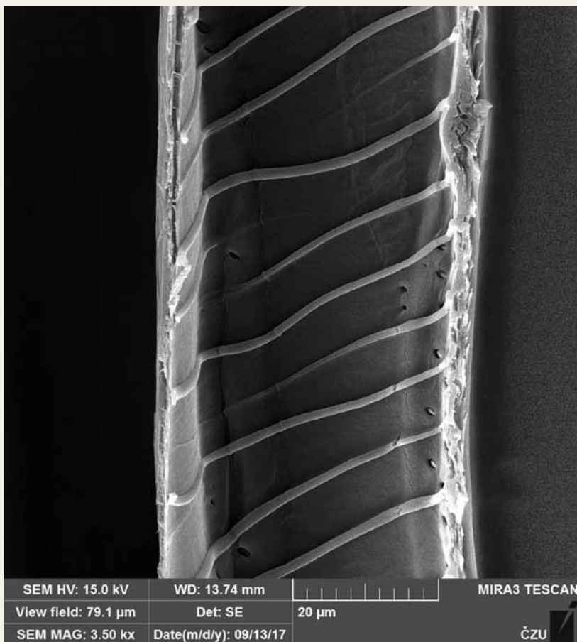
Podélný řez cévou lípy se zřetelně vystupujícími spirálami na vnitřní straně buněčné stěny. Zvětšeno 3 500krát.
