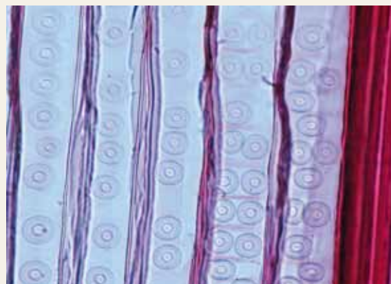
Vzhled dvojteček na stěnách jarních tracheid (radiální řez dřevem modřínu opadavého). Zvětšeno 200krát.
